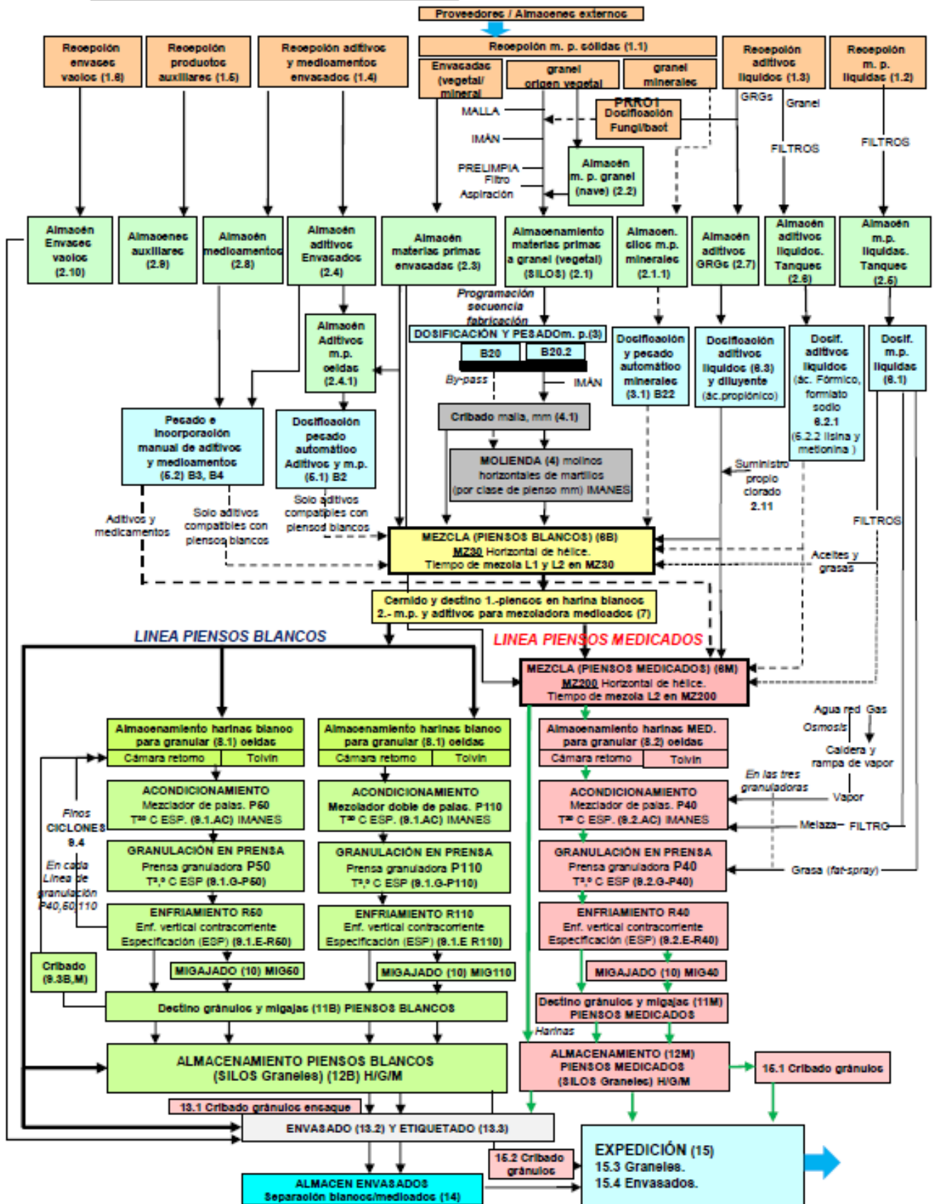
COAVRE - Diagrama de flujo elaboración de los piensos (rev14 22/5/24).
